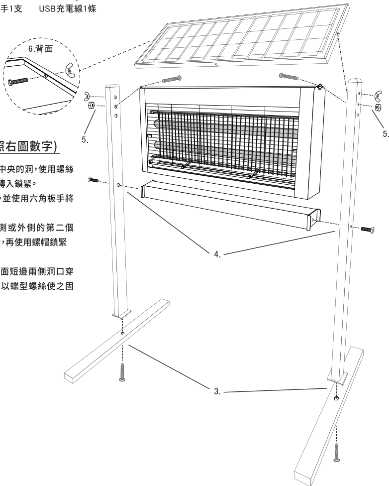
六角板手1支
